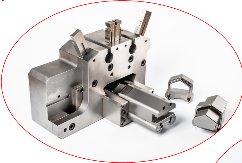
▶ NC Schlitten-Werkzeug
